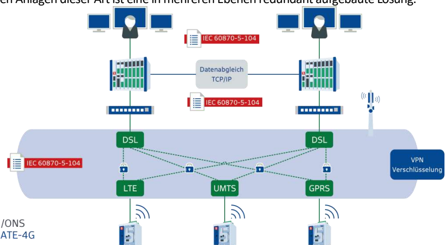
Abbildung 20: M2M-Netzwerk mit redundanten VPN-Verbindungen zu redundantem Fernwirkkopf und Leitsystem
